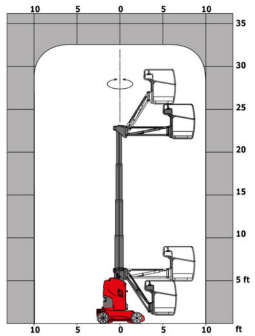
Ábaco de carga para AWP Imperial
